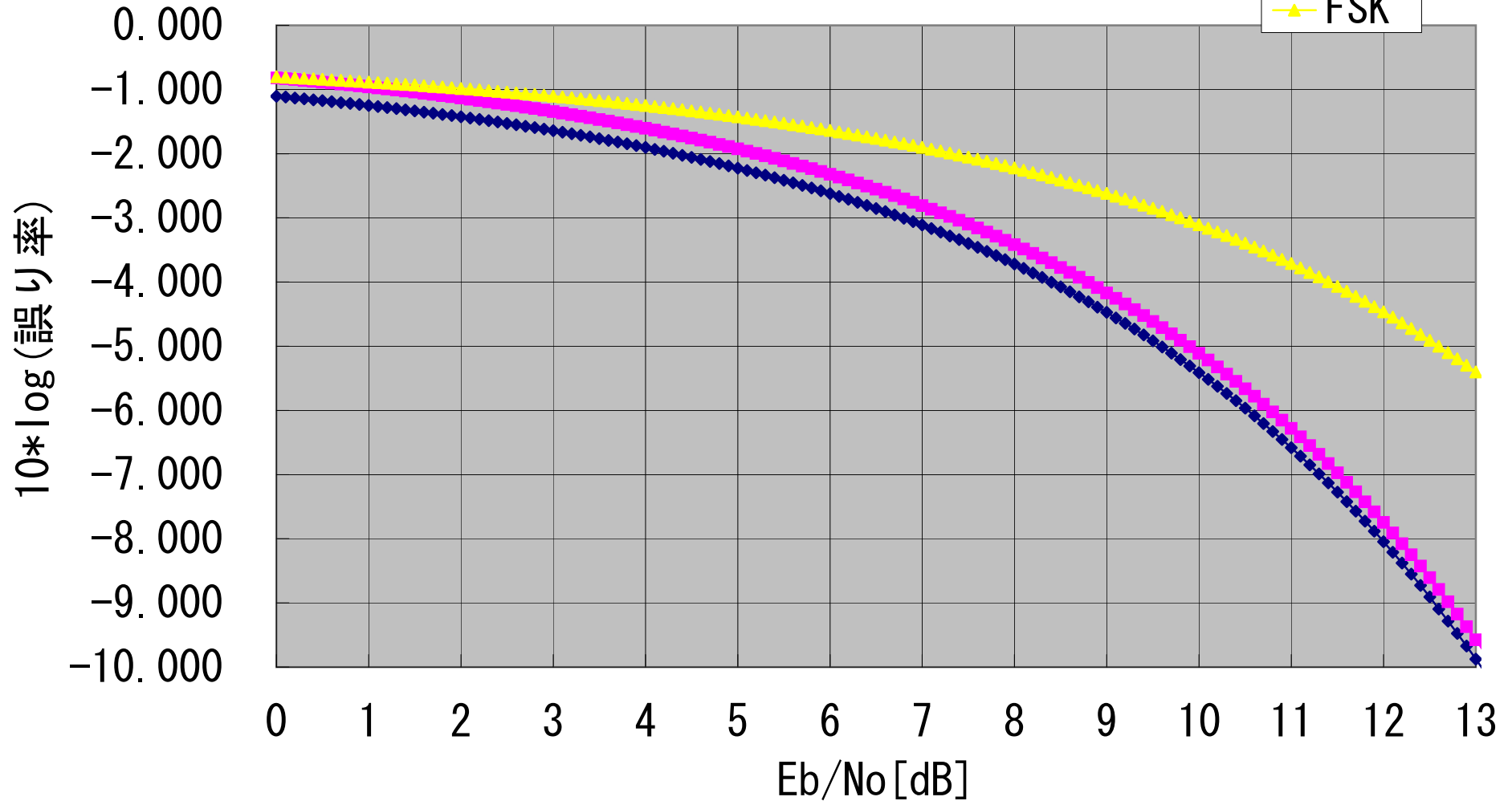
BPSK/QPSKのビット誤り率
